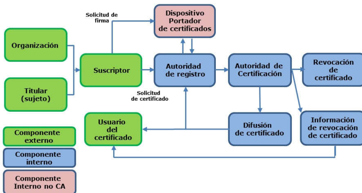
Figura 2 - Diagrama de bloques de las IGC que operan ACs en línea
